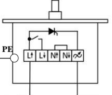
Regulator obrotów REB-1
